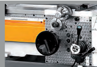
Support-Control Steuerhebel (außer CU 325 RD)
