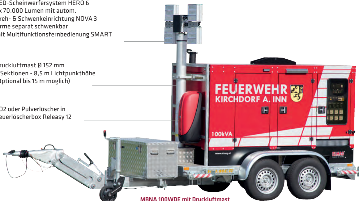
MBNA 100WDE mit Druckluftmast & Dreh- & Schwenkeinrichtung
