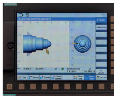
Steuerpanel SIEMENS SINUMERIK 828D
