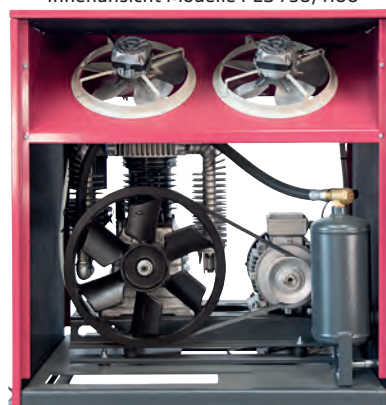
Innenansicht Modelle PLS 750/1100
