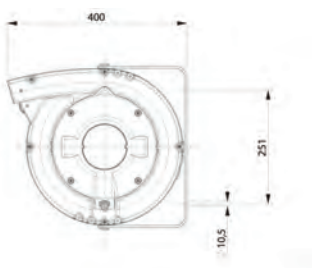
Abmessungen des Modells INDUSTRIE 12
