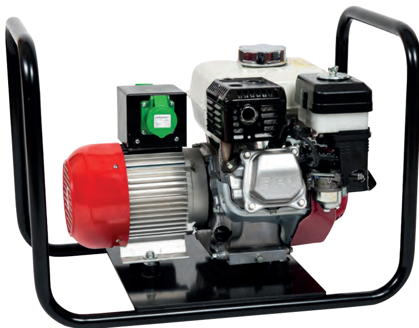
Abb. zeigt HFUM 1,5kVA
