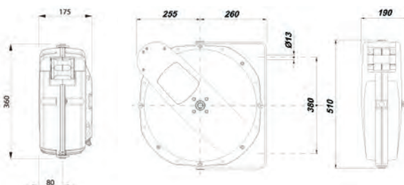
Abmessungen des Modells INDUSTRIE 21
